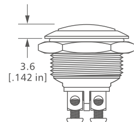
Domed Actuator
