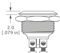
Flat Actuator
